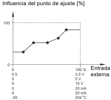
Fig. 49 Tabla de influencia (ejemplo con cinco puntos)
