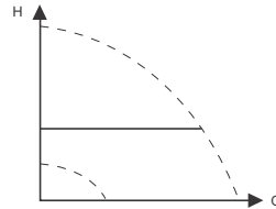
Fig. 26 "Presión constante"
