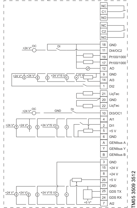
Fig. 8 Terminales de conexión de las bombas CRE, CRIE, CRNE, SPKE y MTRÉ
