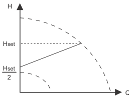
Fig. 25 "Pres. proporcional"
