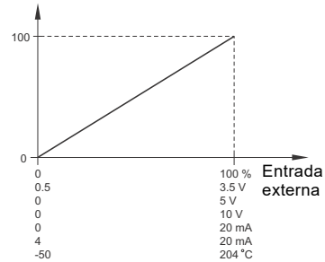
Fig. 47 Función lineal
